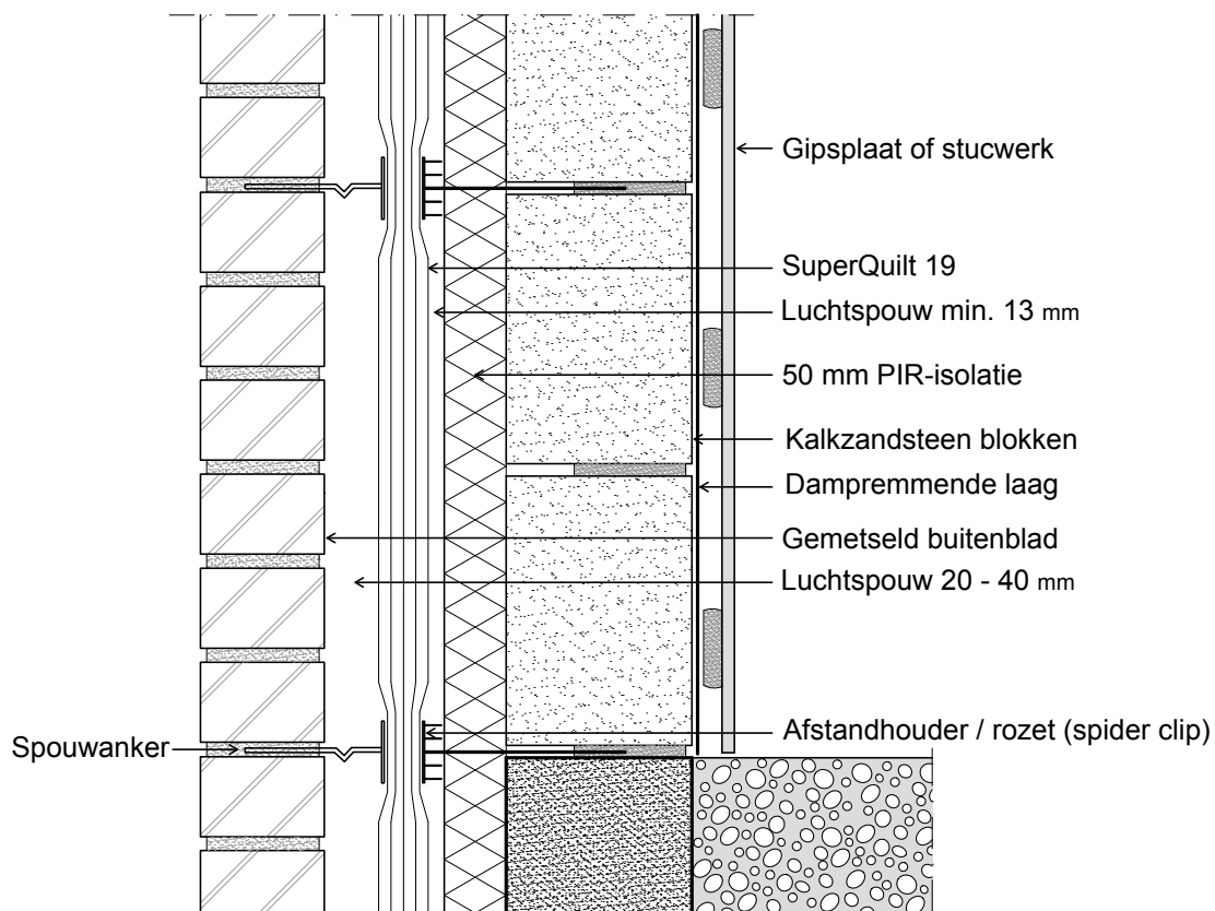
Figuur 2 – Hybride toepassing van SuperQuilt 19 en PIR-schuim in spouwmuur (nieuwbouw)
