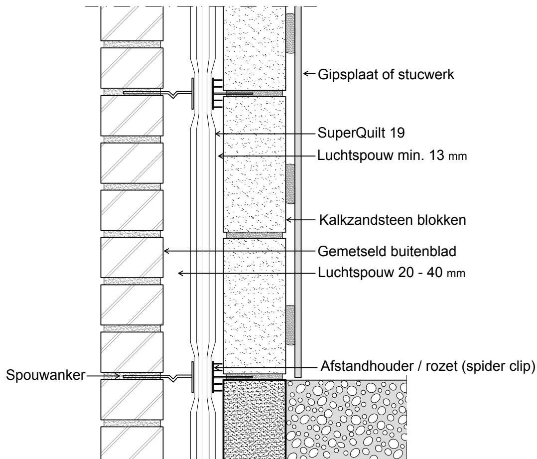
Figuur 1 – Toepassing van SuperQuilt 19 in spouwmuur (nieuwbouw)
