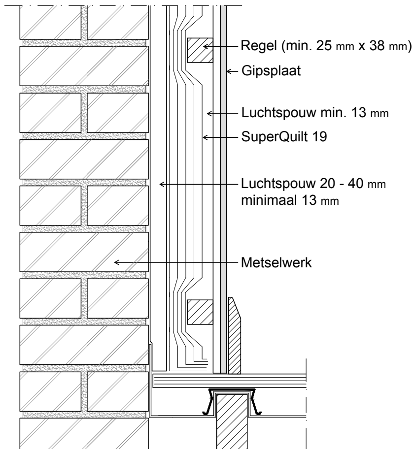
Figuur 3 – Toepassing tegen de binnenzijde van een steens buitenmuur (renovatie)
