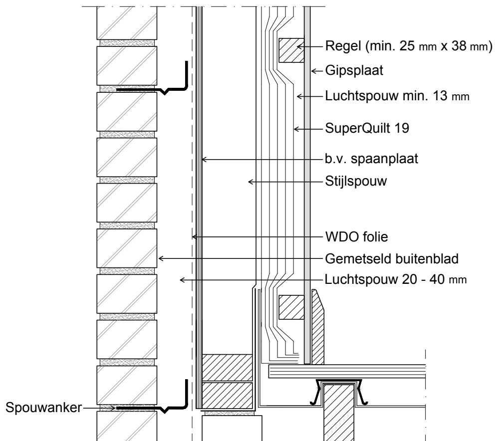
Figuur 4 – Toepassing in houtskeletbouw (nieuwbouw)
